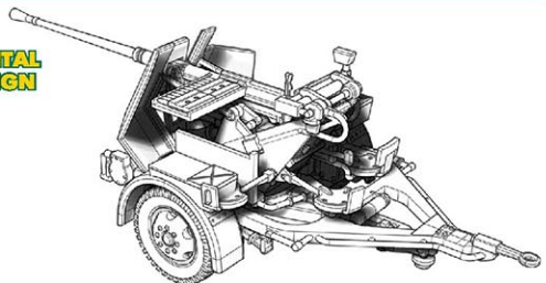
72570 3,7cm Flak 36
